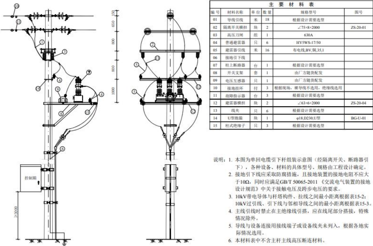
图-15 单回电缆引下杆组装置示意图(经隔离开关、断路器引下)
