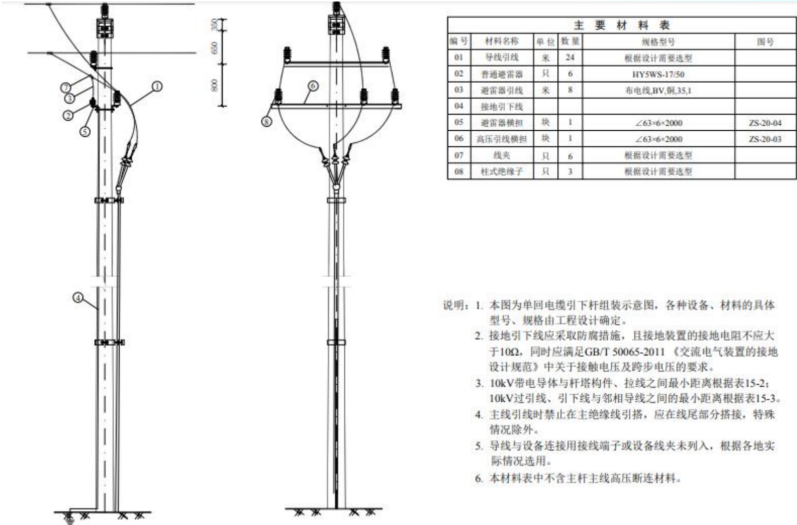
图-13 单回电缆引下杆组装置示意图
