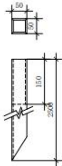
接地极制作示意图
