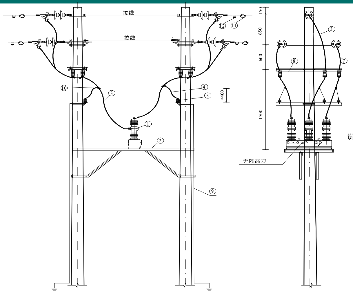
图 15-7-02 单回双杆柱上断路器杆组装机示意图（外加双侧隔离开关\三角排列）
