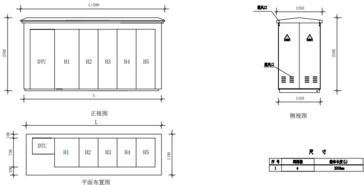
图-3 电气平断面布置图（两进两出）
