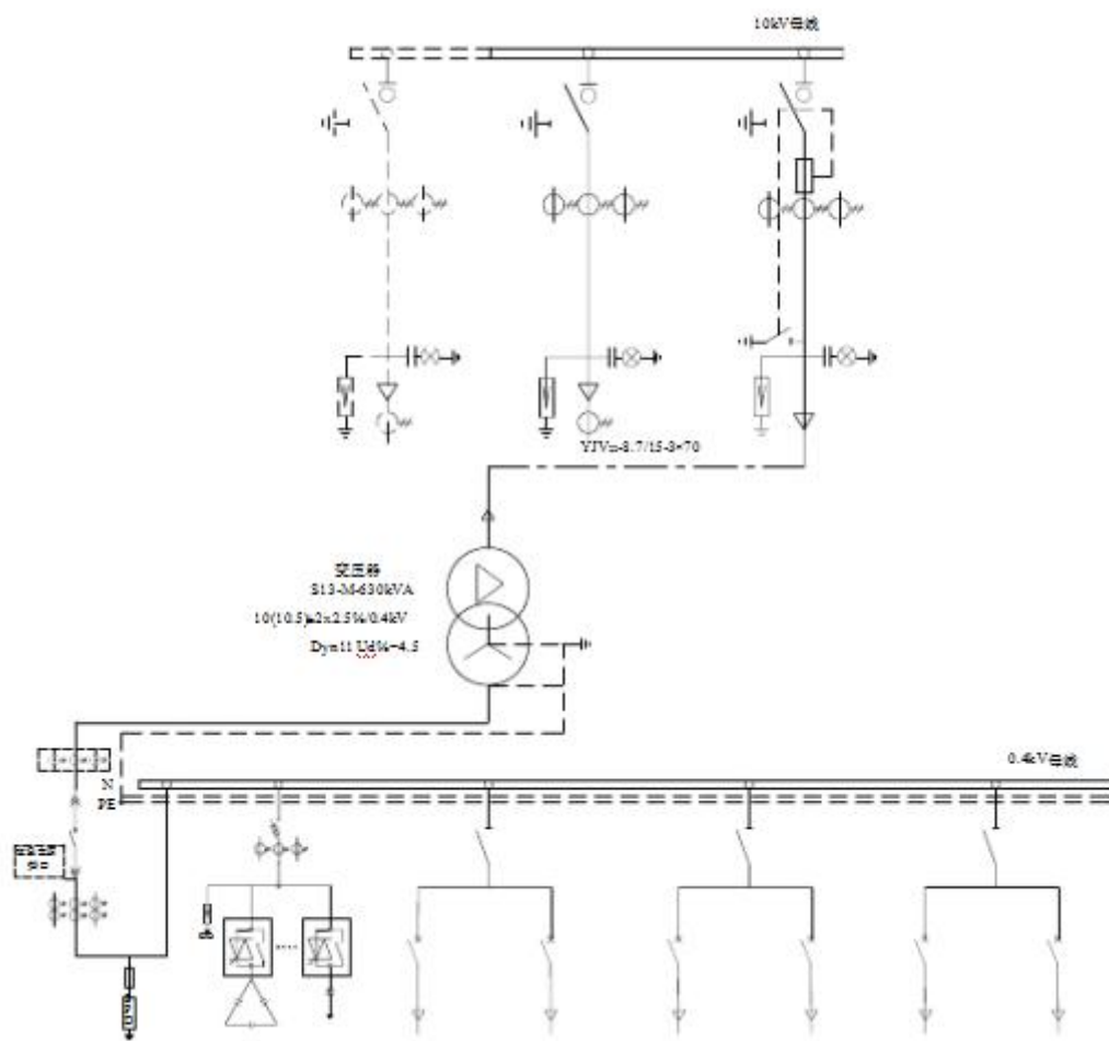
图-3 电气主接线图(630kVA)
